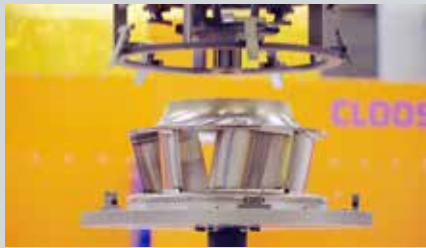
Lüfterrad
